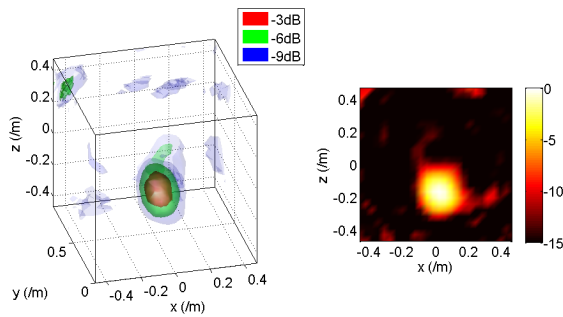
Figure 7. Gauche : Image 3D reconstruite à partir du signal comprimé - Droite : Coupe à une distance de 50 cm.
