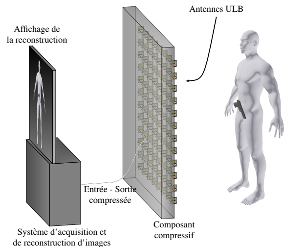
Figure 1. Implémentation d'une technique d'imagerie microonde MIMO ULB compressive appliquée à la détection d'objets enfouis.
