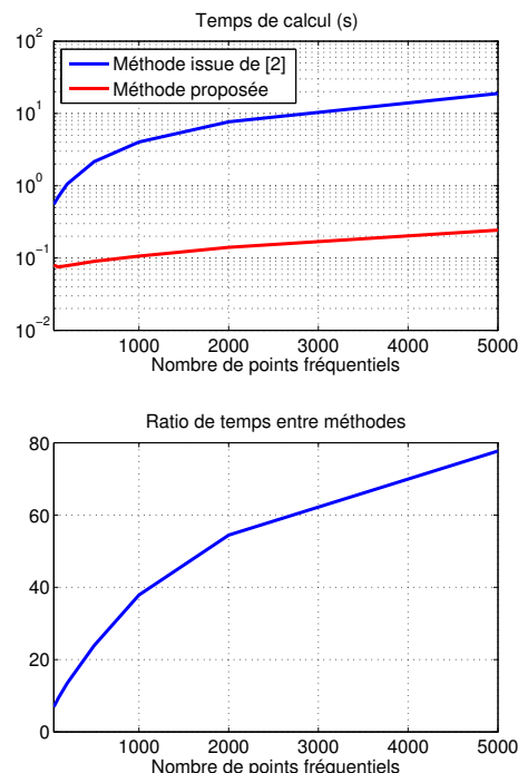
Figure 4. Haut : Temps de calcul des images radar pour chaque méthode en fonction du nombre de points fréquentiels. Bas : Ratio entre les temps de calcul.
