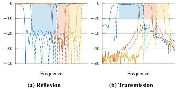
Figure 7: Réponse du triplexeur en dB: circuit (tréma) vs simulation (points) vs measurements (continue).
