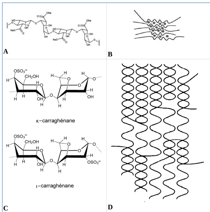
Formules moléculaires des alginates (A) et des carraghénanes (C), et schéma représentatif de leurs structures, respectivement « en boîte à œufs » (B) et « en double hélice » (D). Schéma (B) d'après X.Y. He et al. , RSC Adv. , 2016, 6, p. 114779 (© Royal Society of Chemistry, 2016); schéma (D) d'après R.P. Millane et al. , Carbohydr. Res. , 1988, 182, p. 1 (© Elsevier, 1988).
