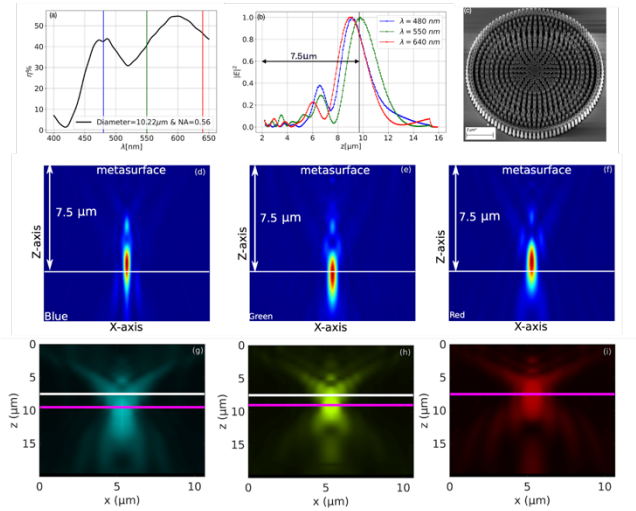
Fig. 1 Optimized RGB metalens
