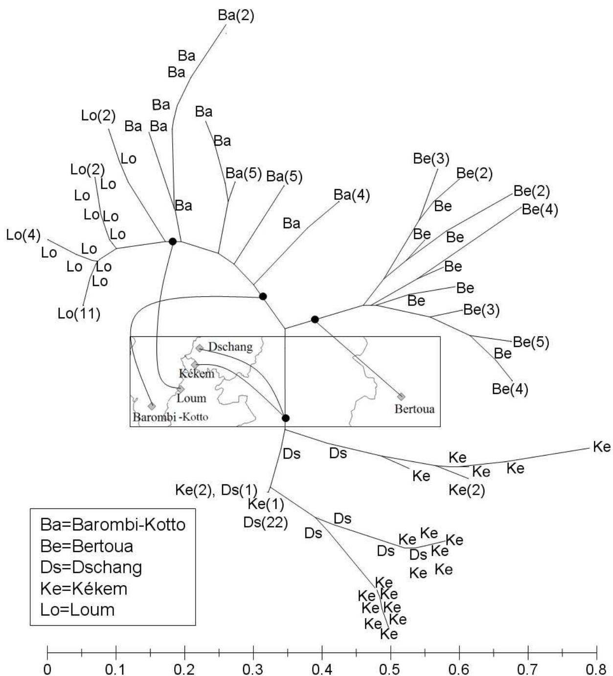
Figure 12 : Arbre de divergence des échantillons de B. truncatus récoltés en septembre-octobre 2009. Le nombre de génotypes multilocus est indiqué entre parenthèses.
